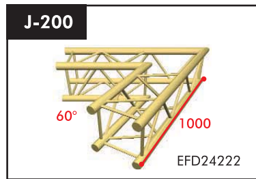
2 Wege Ecke 60° Gewicht: 5,30kg Preis: 253,50 €
