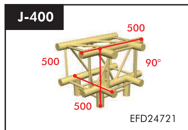
4 Wege T-Stück 90° Gewicht: 4,50kg Preis: 398,70 €
