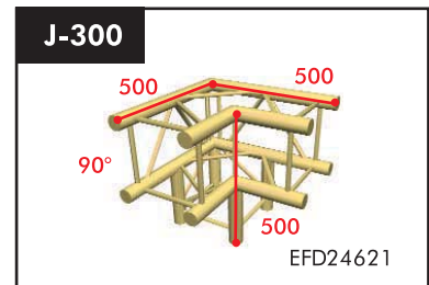
3 Wege Ecke 90° Gewicht: 4,00kg Preis: 291,70 €
