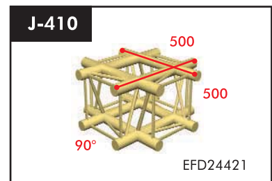
4 Wege Kreuz 90° Gewicht: 4,50kg Preis: 398,70 €
