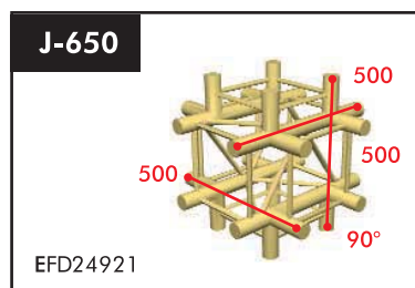
6 Wege T-Stück 90° Gewicht: 5,30kg Preis: 524,90 €
