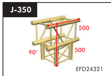
3 Wege T-Stück 90° Gewicht: 4,00kg Preis: 291,70 €
