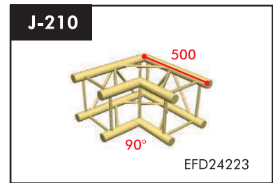
2 Wege Ecke 90° Gewicht: 2,90kg Preis: 225,50 €
