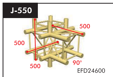
5 Wege T-Stück 90° Gewicht: 5,00kg Preis: 479,00 €
