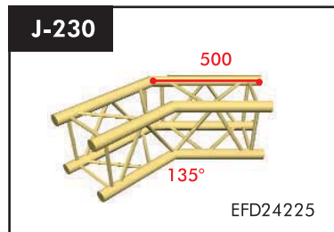
2 Wege Ecke 135° Gewicht: 2,90kg Preis: 225,50 €
