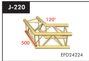
2 Wege Ecke 120° Gewicht: 2,90kg Preis: 225,50 €
