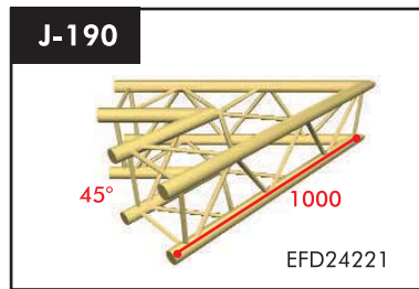
2 Wege Ecke 45° Gewicht: 3,50kg Preis: 253,50 €
